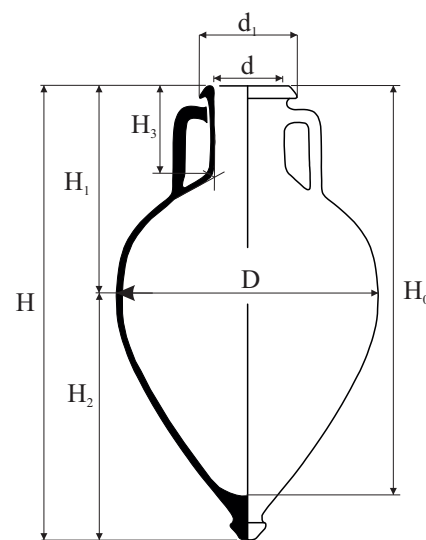
Рис. 7. Схема замеров параметров амфоры
